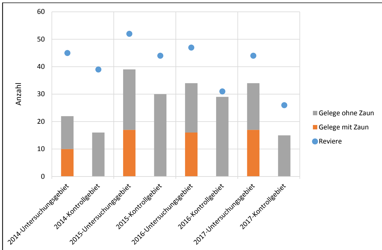
Abb. 5: Anzahl der Brachvogel Reviere, sowie Gelege (mit und ohne Zaun) der Untersuchungs- und Kontrollgebiete der Jahre 2014 - 2017.
