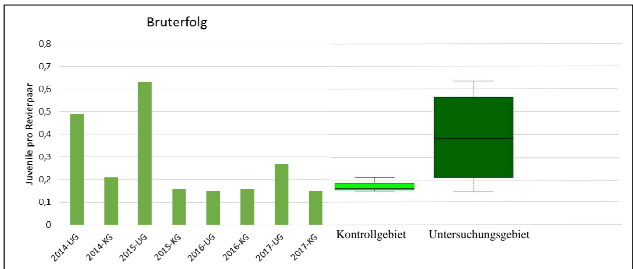
Abb. 8: Bruterfolg (flügge Juvenile pro Revierpaar und Jahr) beim Großen Brachvogel in der ETS. Links: während der Untersuchungsjahre 2014 - 2017 innerhalb der Untersuchungs- (UG) und der Kontrollgebiete (KG). Rechts: Boxplot der Überlebensrate in den Kontroll- und Untersuchungsgebieten für alle Jahre zusammengefasst (n = 4). Boxplot Erklärung s. Abb. 6.
